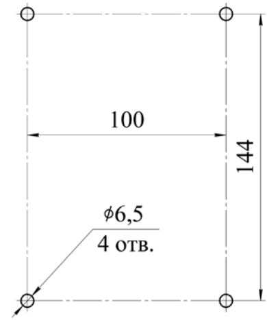
Рисунок 5 - ГППТ-1,0(тр)
